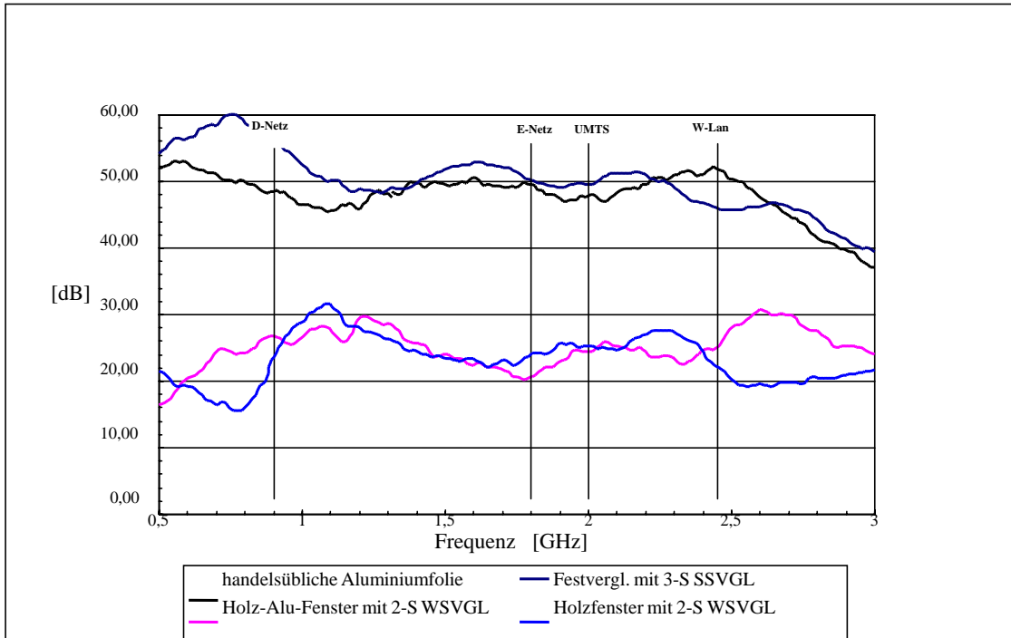
Abb. 8: Schirmdämpfung von 2-Scheiben-Wärmeschutzverglasung und 3-Scheiben-Sonnenschutzverglasung
