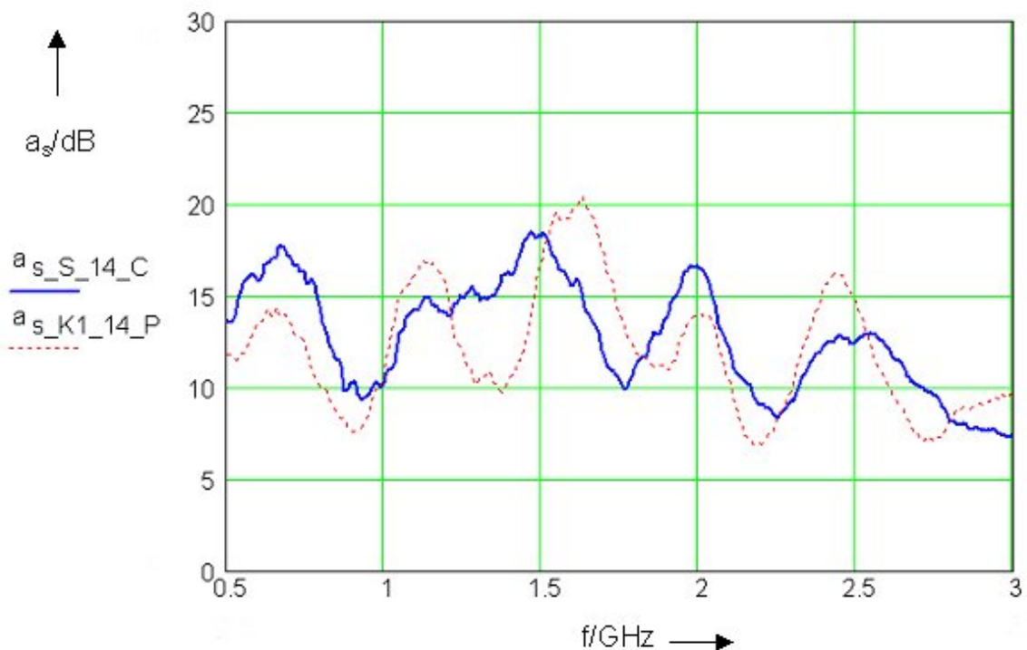
Abb. 20: Schirmdämpfung im Schlafzimmer von Typ „C“ und im Kinderzimmer 1 von Typ „P“ (jeweils Dachgeschoss, gleiche räumliche Zuordnung).
