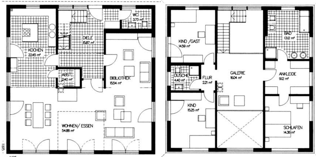
Abb. 11: Grundriss von Typ „P“.
